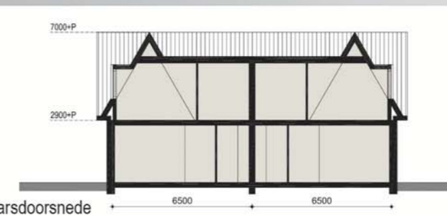
dwarsdoorsnede
