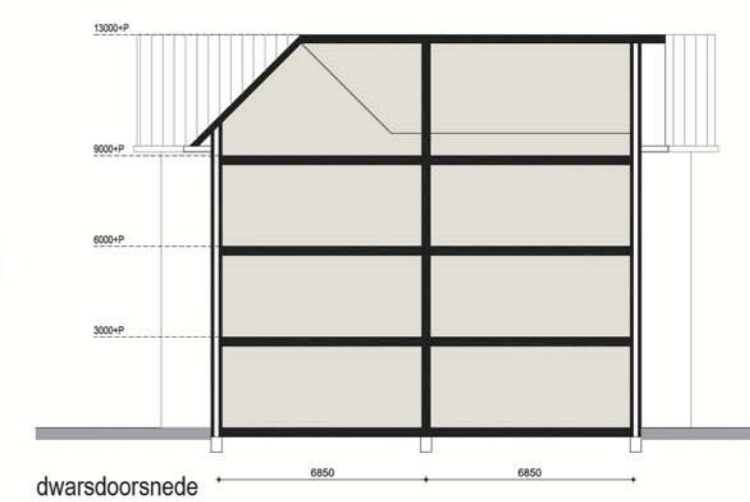
dwarsdoorsnede
